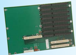
7 ISA/2 PCI
